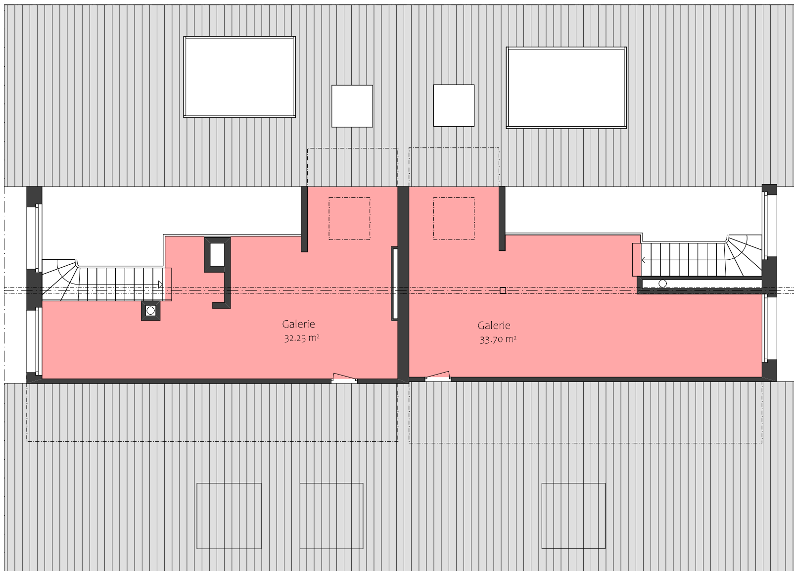
Lehnstrasse 103 / Galerie Mst.: 1:100
