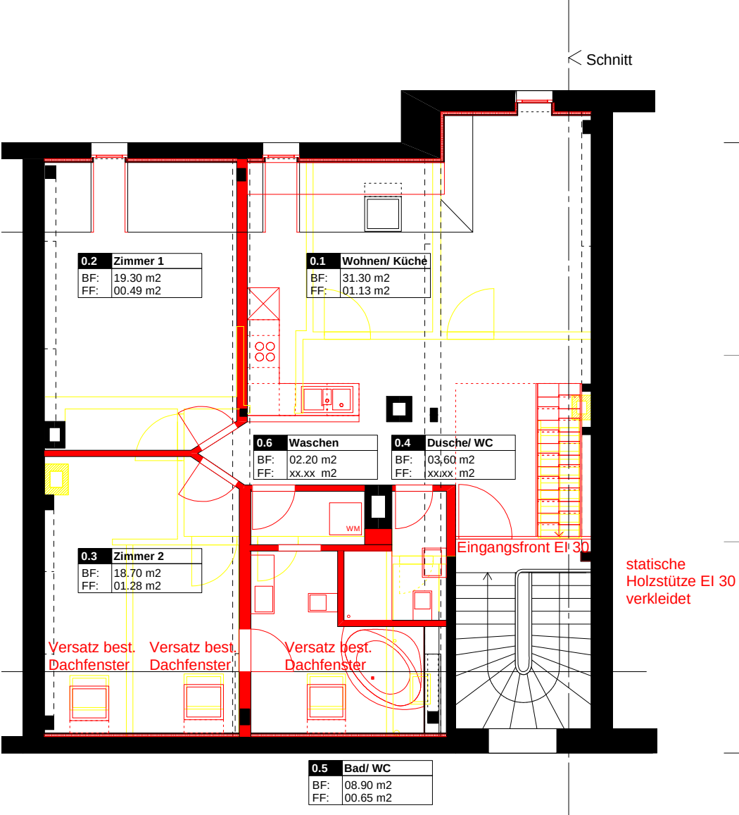
Grundriss Dachgeschoss 1_ Mst: 1/100
