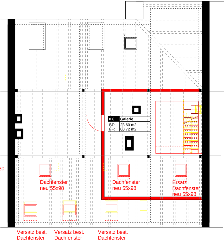
Grundriss Dachgeschoss 2_ Mst: 1/100
