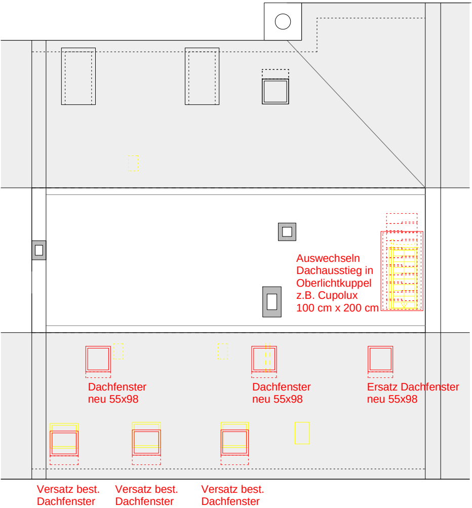
Aufsicht Dachterrasse_ Mst: 1/100
